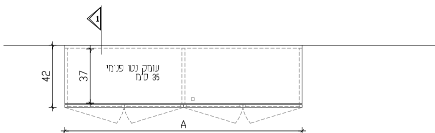
חלק 1-1
